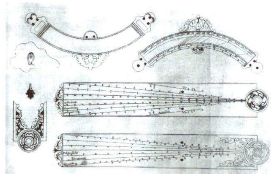
Fig. 3. Il compasso geometrico e militare di Galileo Galilei, in Opere di Galileo Galilei , cit., tavola fuori testo dopo p. CXII, 19x36,5 cm.
